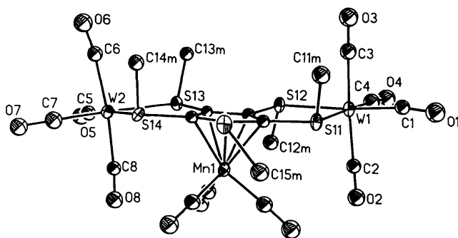
Abb. 2. Molekülstruktur von 4
