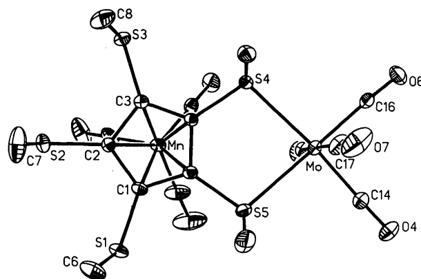
Abb. 1. Molekülstruktur von 3
