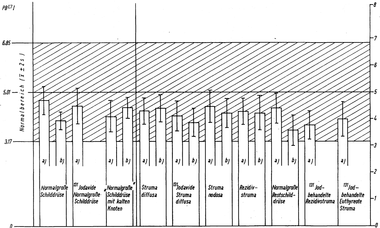
Abb. 2: Mittlere PB^{127}I -Werte ( \bar{x} \pm s ) bei Strumapatienten: a) mit kontinuierlicher Speicherungszunahme bzw. Plateaukurve und b) mit beschleunigtem Radiojodumsatz.
