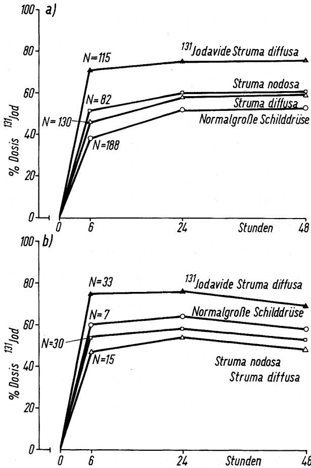
Abb. 1: 131 Jod-Speicherung a) bei Patienten mit kontinuierlicher Speicherungs Zunahme bzw. Plateaukurve und b) bei Patienten mit beschleunigtem thyreoidalem 131 Jodumsatz. Angegeben sind die Mittelwerte ( \bar{x} ) für normalgroße Schilddrüsen (○—○), diffuse Strumen (△—△), Knotenstrumen (□—□) und 131 Jod-averse diffuse Strumen (▲—▲), die dazugehörigen Standardabweichungen sind aus Tab. 1 zu entnehmen.
