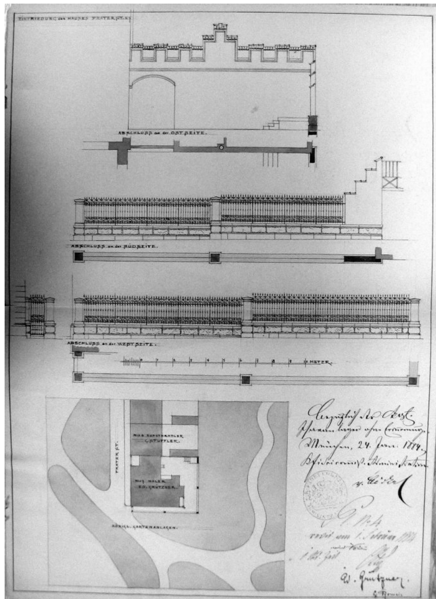
Abbildung 60: Grützner-Haus, Plan der Einfriedung und Situationsplan, Leonhard Romeis, 1884.
