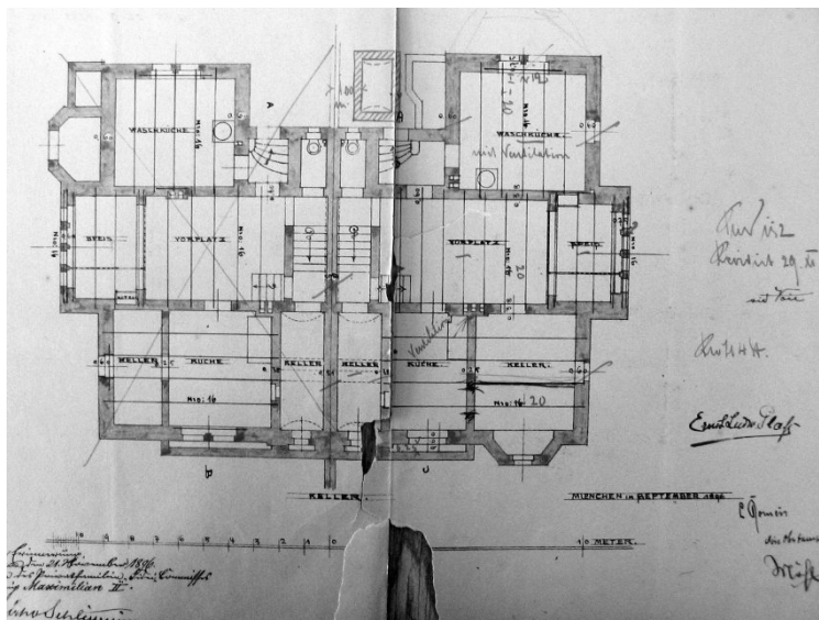
Abbildung 75: Doppelvilla Plaf/Kerschensteiner, Grundriß Kellergeschoß, Leonhard Romeis, 1896, Plan nach Westen ausgerichtet.
