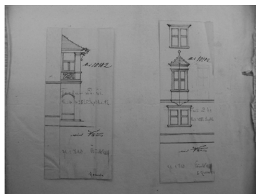
Abbildung 24: Grünzner-Haus, Tekturen Westseite, Leonhard Romeis.
