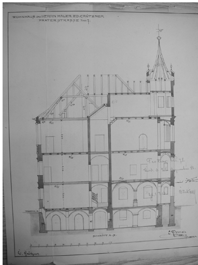
Abbildung 36: Grütznerturm, Schnitt A-B, Leonhard Romeis, 1882.
