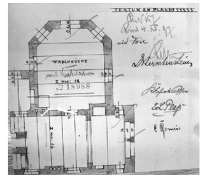
Abbildung 76: Doppelvilla Plaf/Kerschensteiner, Grundriß Kellergeschoß: Tektur, Leonhard Romeis, 1896.
