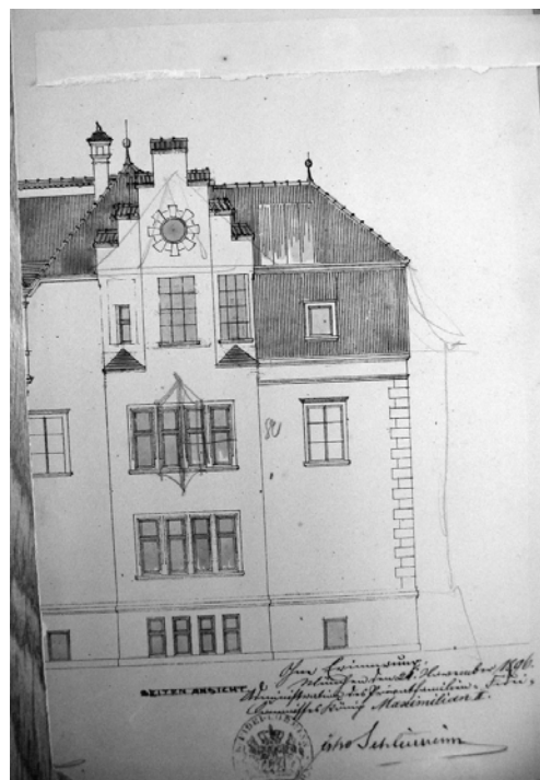
Abbildung 68: Doppelvilla Plaß/Kerschensteiner, Nordseite, Leonhard Romeis, 1896.
