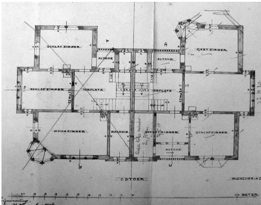
Abbildung 78: Doppelvilla Pläß/Kerschensteiner, Grundriß erster Stock, Leonhard Romeis, 1896, Plan nach Westen ausgerichtet.
