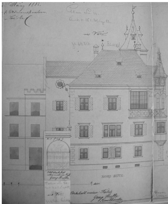
Abbildung 16: Grützner-Haus, Ansicht Nordseite, Leonhard Romeis, 1882.
