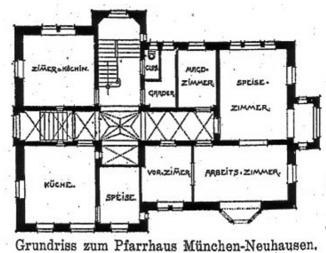
Abbildung 104: Katholisches Pfarrhaus Neuhausen. Grundriß Erdgeschoß, Plan nach Süden ausgerichtet, publiziert 1905.
