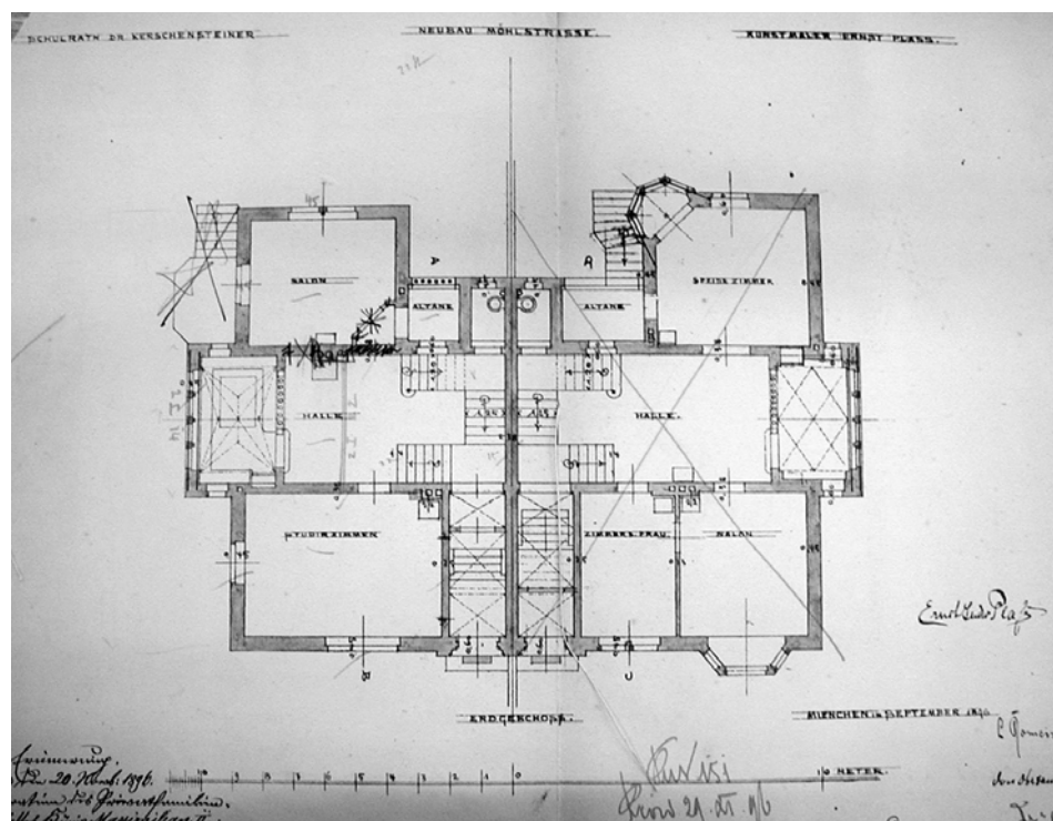
Abbildung 77: Doppelvilla Plaf/Kerschensteiner, Grundriß Erdgeschoß, Leonhard Romeis, 1896, Plan nach Westen ausgerichtet.
