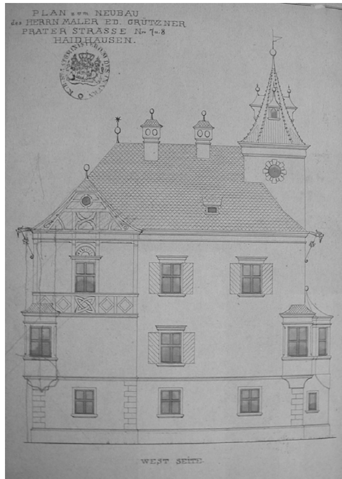
Abbildung 23: Grünzner-Haus, Ansicht Westseite, Leonhard Romeis, 1882.
