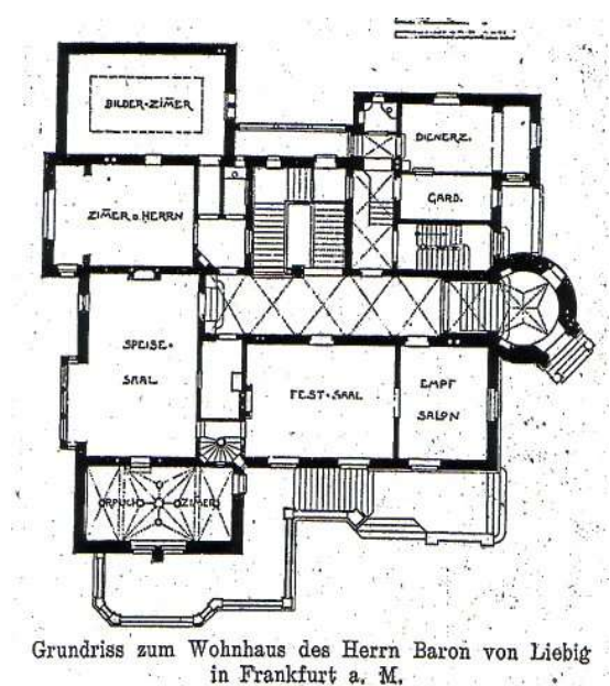
Abbildung 8: Villa für Heinrich von Liebig, Frankfurt am Main, Leonhard Romeis, 1888-1902, Grundriß Erdgeschoß.
