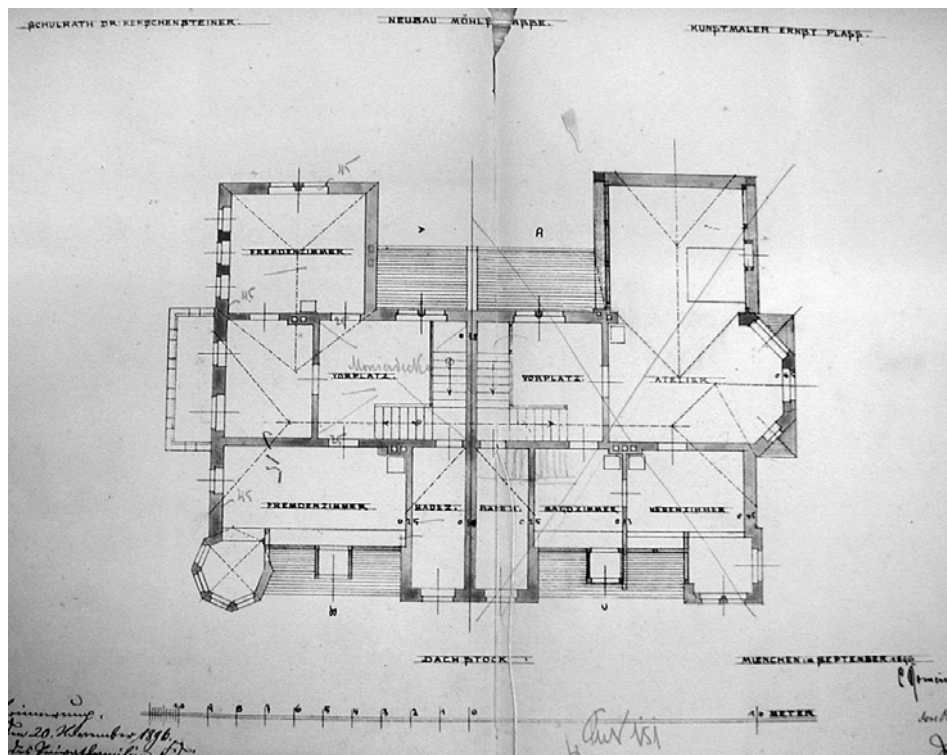
Abbildung 80: Doppelvilla Pläß/Kerschensteiner, Grundriß Dachstock (zweiter Stock), Leonhard Romeis, 1896, Plan nach Westen ausgerichtet.
