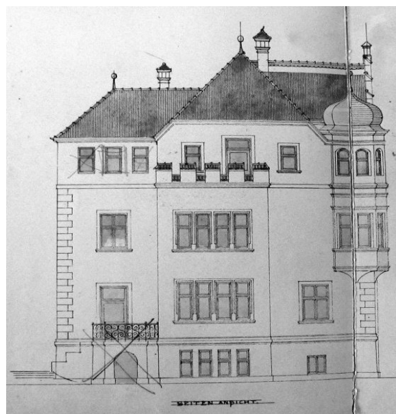
Abbildung 70: Doppelvilla Plaß/Kerschensteiner, Südseite, Leonhard Romeis, 1896.
