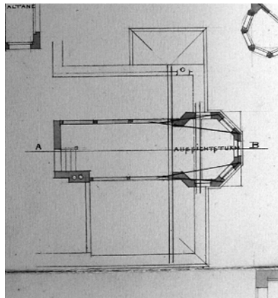
Abbildung 35: Grütznerturm, Grundriß Turmgewölb, Leonhard Romeis, 1882.
