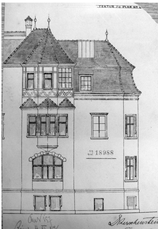
Abbildung 69: Doppelvilla Plaß/Kerschensteiner, Nordseite: Tektur, Leonhard Romeis, 1896.
