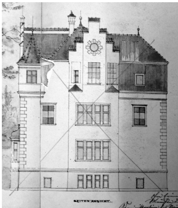
Abbildung 67: Doppelvilla Plaß/Kerschensteiner, Nordseite, Leonhard Romeis, 1896.
